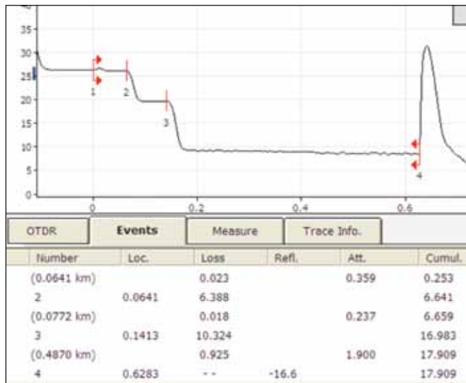
Ilustración 3. Utilizando una amplitud de pulso con un rango dinámico suficiente, un técnico con experiencia puede medir la pérdida de extremo a extremo.
