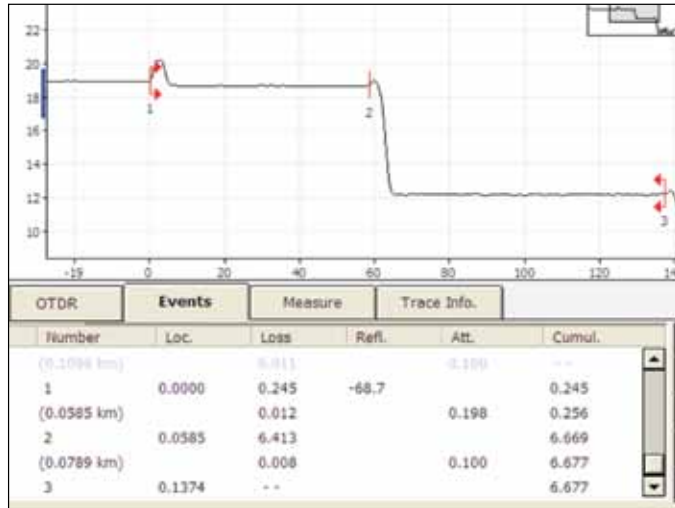
Ilustración 2. Utilizando una amplitud de pulso más larga que para la primera curva, un técnico experimentado califica el área del divisor y posiblemente la parte entre dos divisores. En función de los resultados, el técnico podría tener que repetir este segundo paso para encontrar el pulso óptimo para medir la pérdida del divisor.
